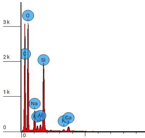
Elementspektrum KMF 2513956-01
