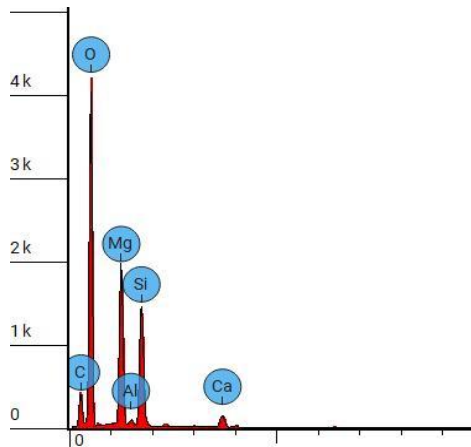
Elementspektrum Chrysotil 2513956-02
